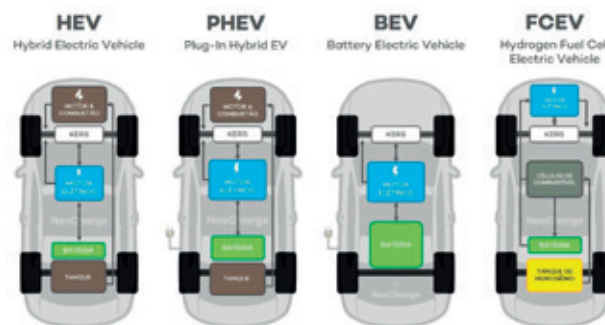
Figura 1. Comparativo de tipos de powertrain eletrificados. Fonte: Neocharge.
